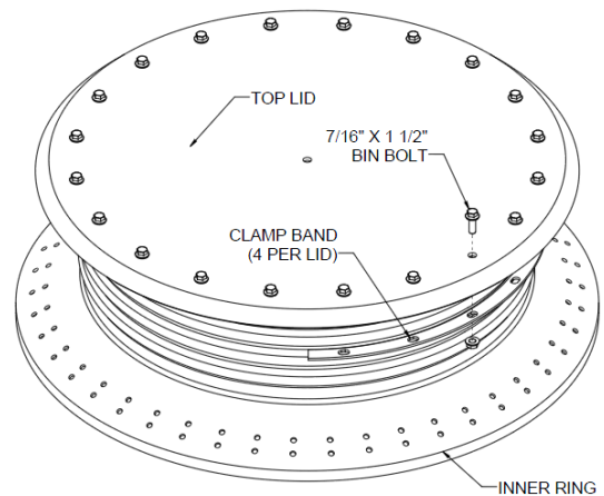
9806779 - BN LID-TOP 30"HD ASY PNT TLAP-30 GRY
